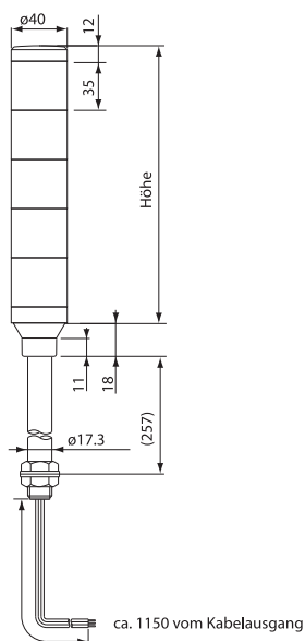
Typ LCS
