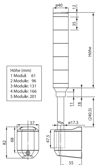
Typ LCS-K
